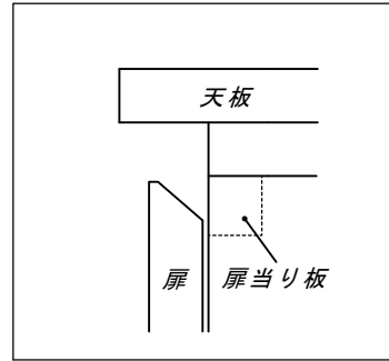
扉手掛け詳細図
