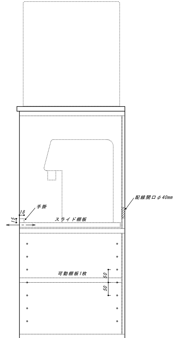
【側面図】
