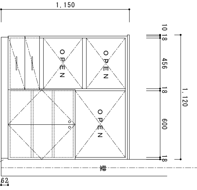
正面図 1 : 20
