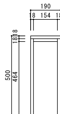
【正面図】
