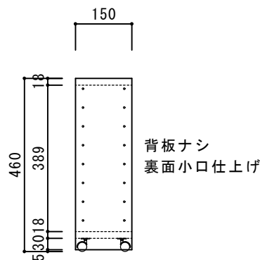
【横断面図】
