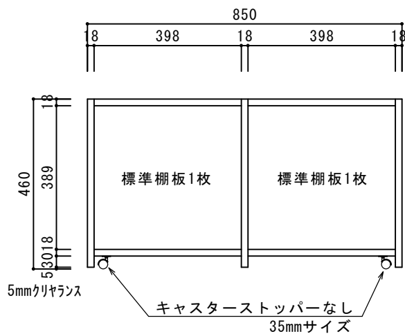
【正面図】
