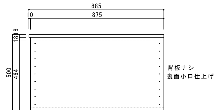
【横断面図】
