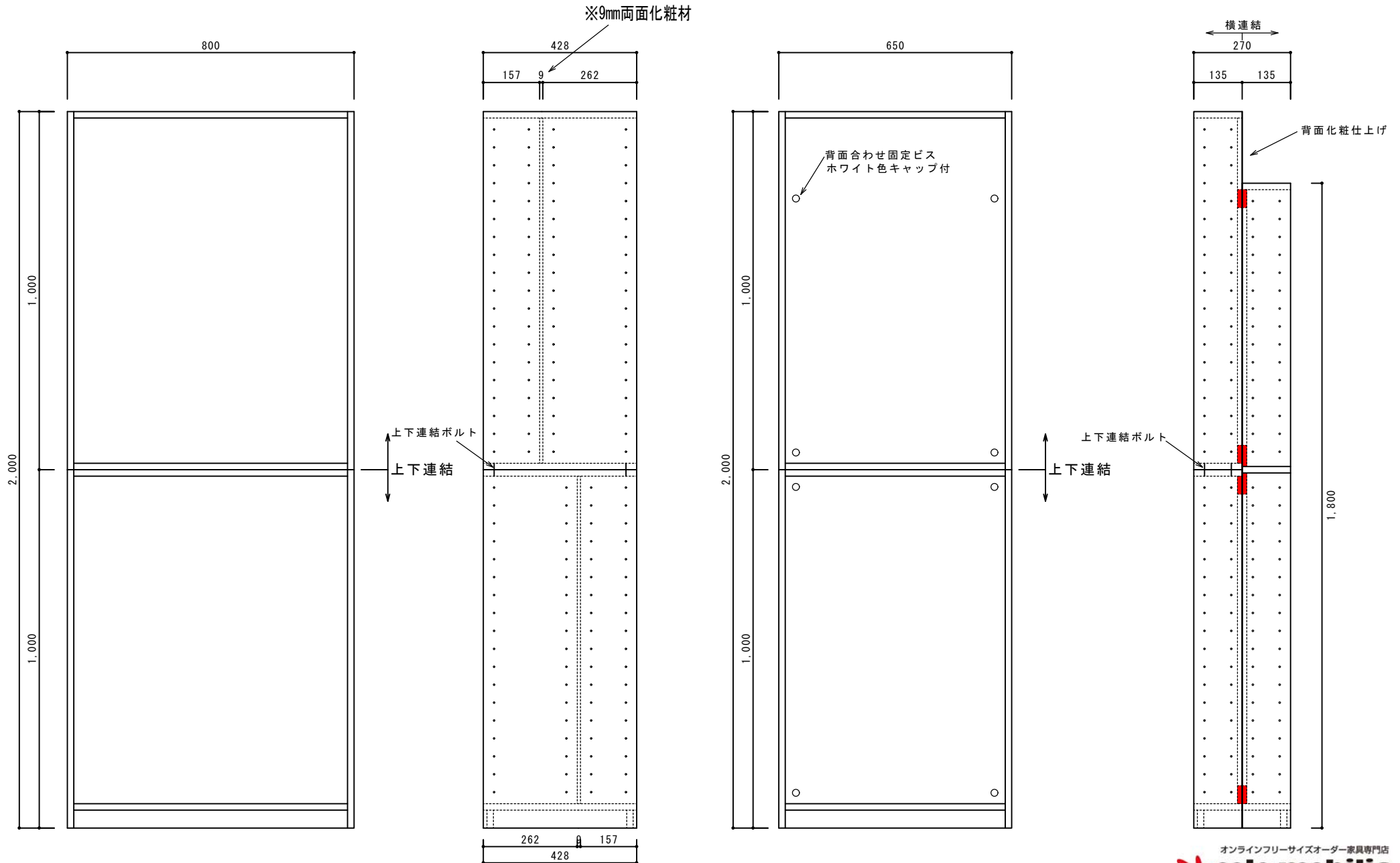
【正面図】
