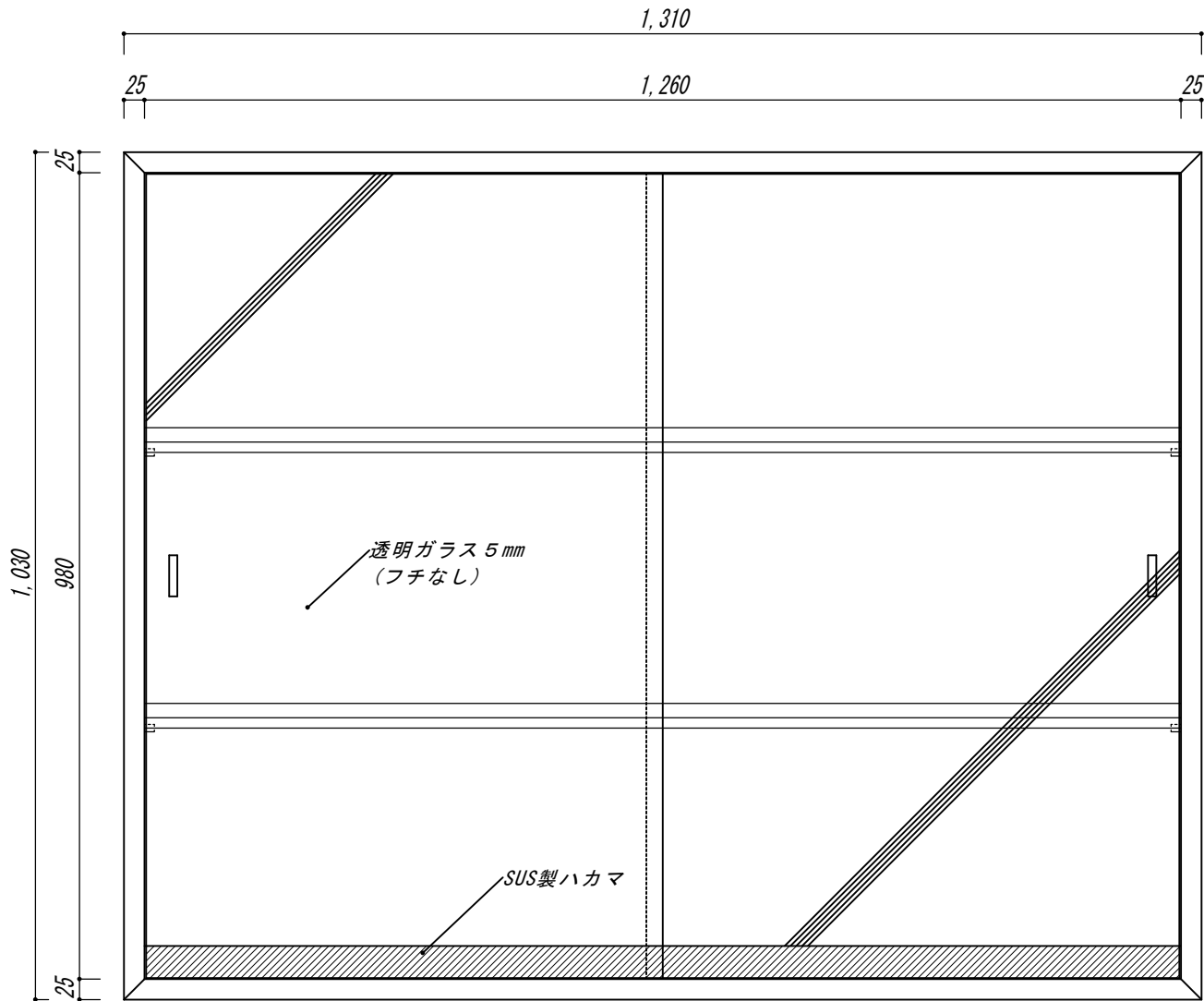
【正面側図】
