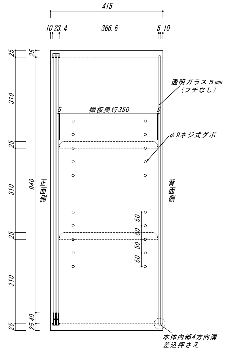
【側面図】
