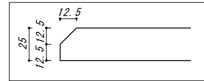
【側面図】
