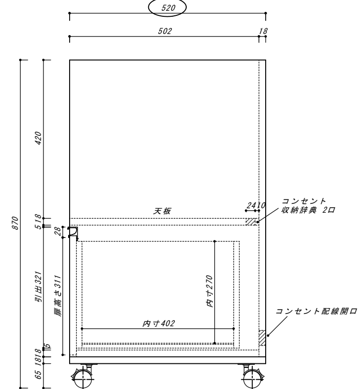
【側面図】
