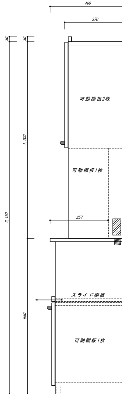
【正面右側面図】
