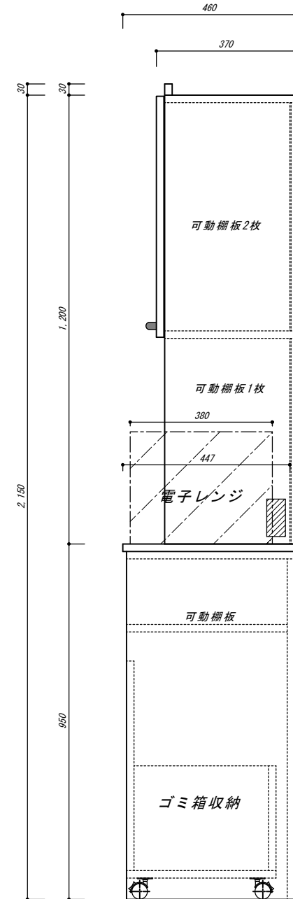
【正面左側面図】
