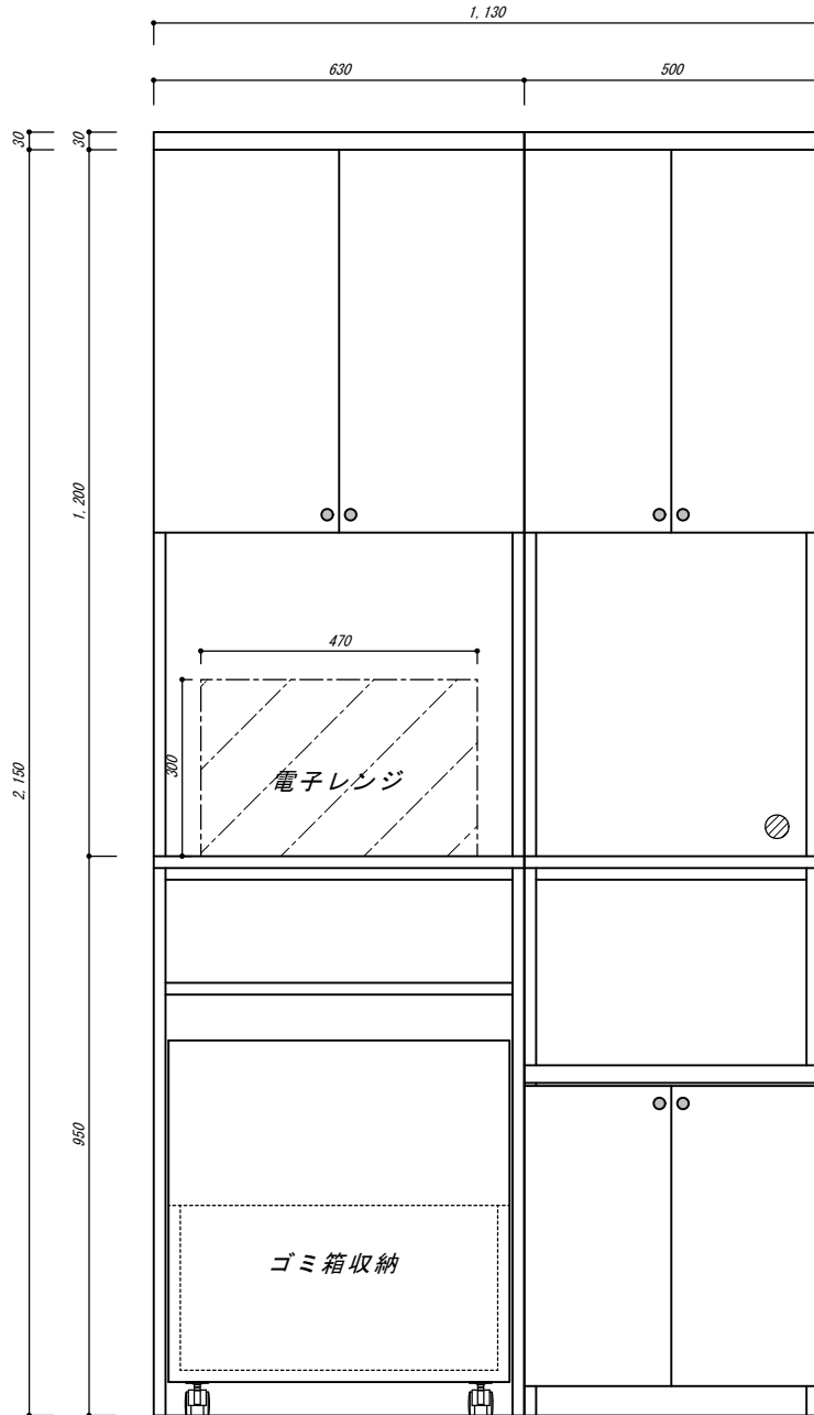
【正面図】
