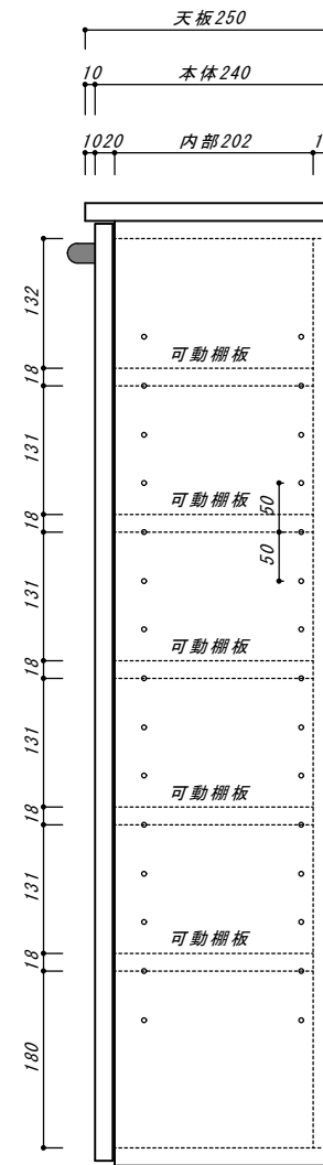
【下足入側面図】
